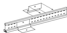
Универсальная клипса для крепления перегородок, используемая с подвесной системой Silhouette
