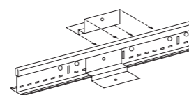
Универсальная клипса крепления перегородок, используемая с подвесной системами Prelude 15 или Prelude 24
