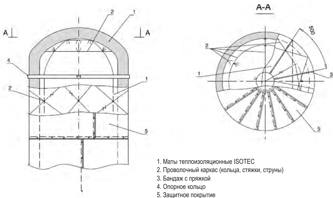
Рисунок 3. Изоляция вертикальных аппаратов матами ISOTEC с креплением проволочным каркасом и металлическим защитным покрытием
