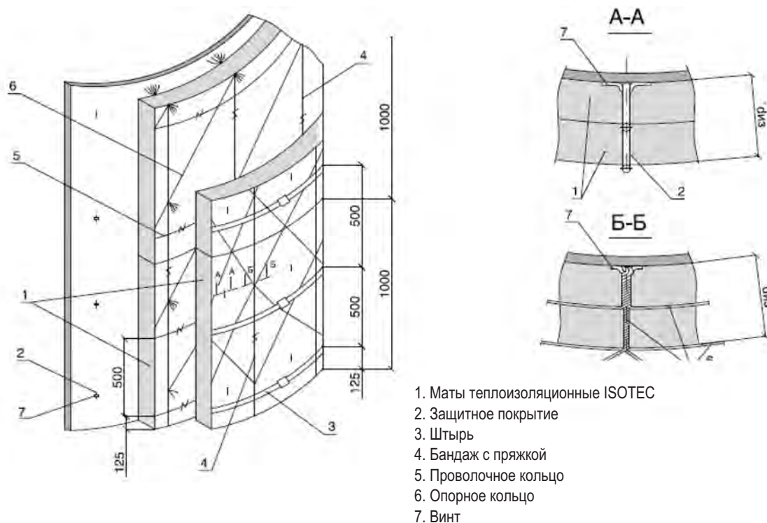
Рисунок 2. Изоляция вертикальных аппаратов матами ISOTEC в два слоя с креплением штырями и стяжками
